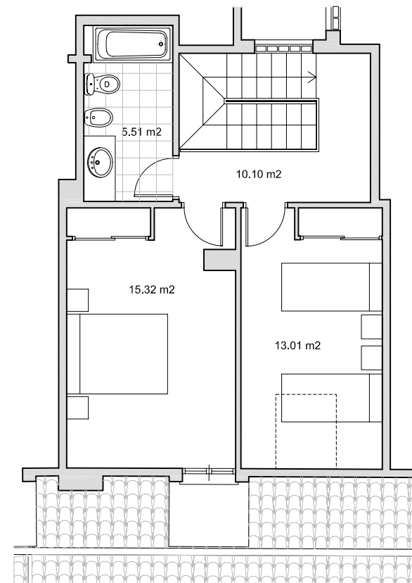
PLANTA BAJO CUBIERTA
